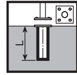
FL4A FL4B Flanschbefestigung Flangia di fissaggio Ø 150 Ø 200 L = 300 L = 300 L = 400 L = 400 L = 500 L = 500
