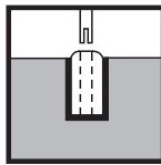
EB150BE Bodenhülse in Fundament Tubo fodera in fondazione
